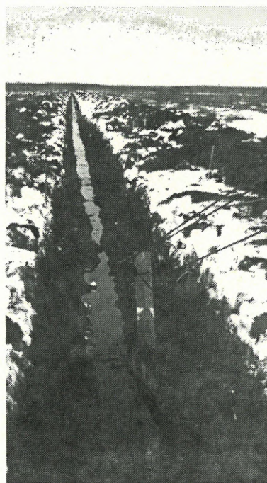
Turpeentuotantoon ojitettavan suon syvät peruskuivatusojat tehdään kaivukoneella.
