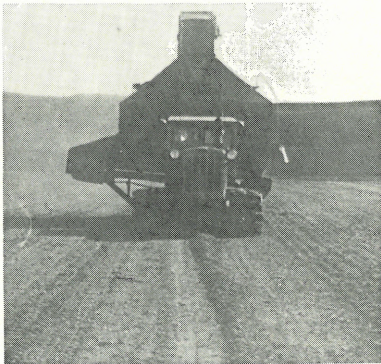
Traktorin vetämä kokoojavaunuun kytketty kuppielevaattori nostaa turpeen vaunun säiliöön.
