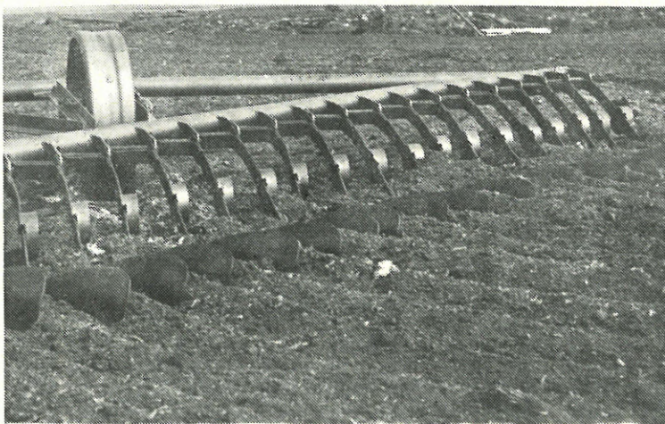
Jyrsinturpeen kääntäjässä on toimivina eliminä rivi pieniä auroja.
