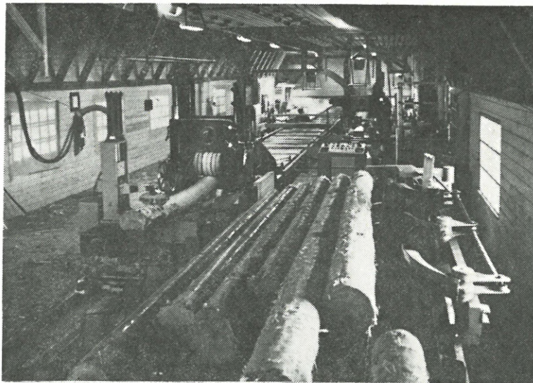
Sahauslinja, jolla puuhun kosketaan käsin vasta kun se on lautoina ja lankkuina.
