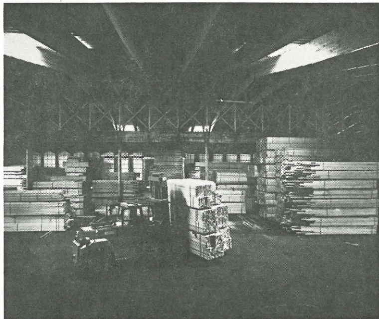
Kuivan tavaravaroitus satamassa. Trukki käsittelee 20–30 kiintom 3 nippuja.
