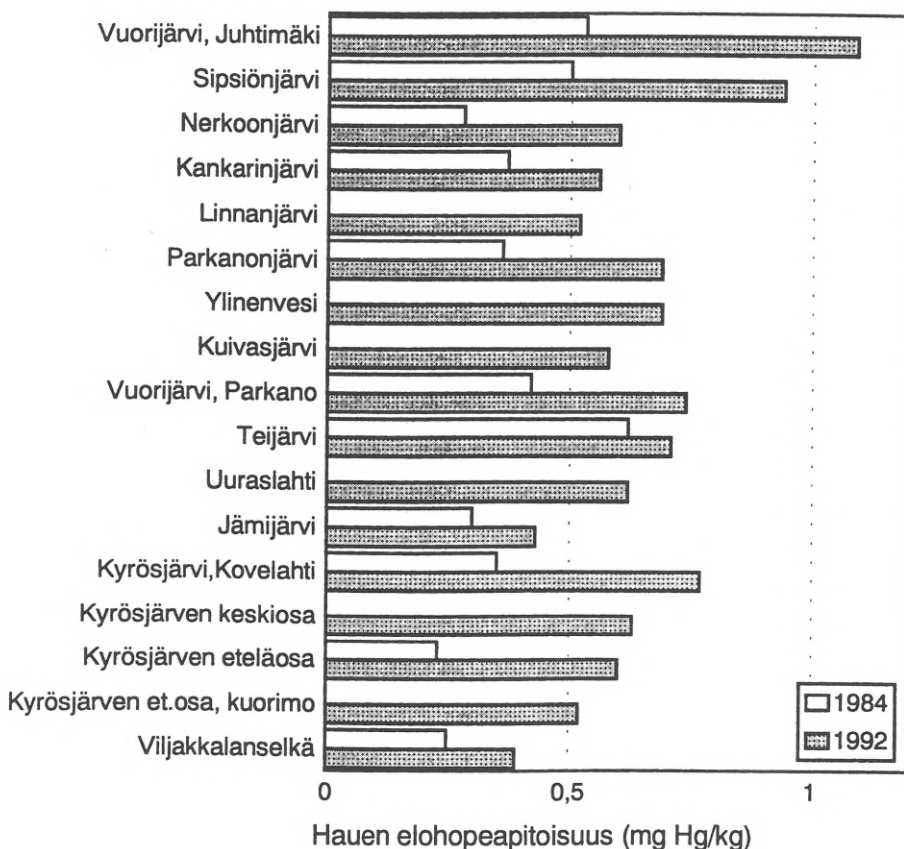
Hauen elohopeapitoisuudet eräissä Parkanon ja lähikuntien järvissä vuosina 1984 ja 1992. (Lähde: Kyrösjärven, Parkanonjärven ja Jämijärven vesiensuojelusuunnitelma.)
