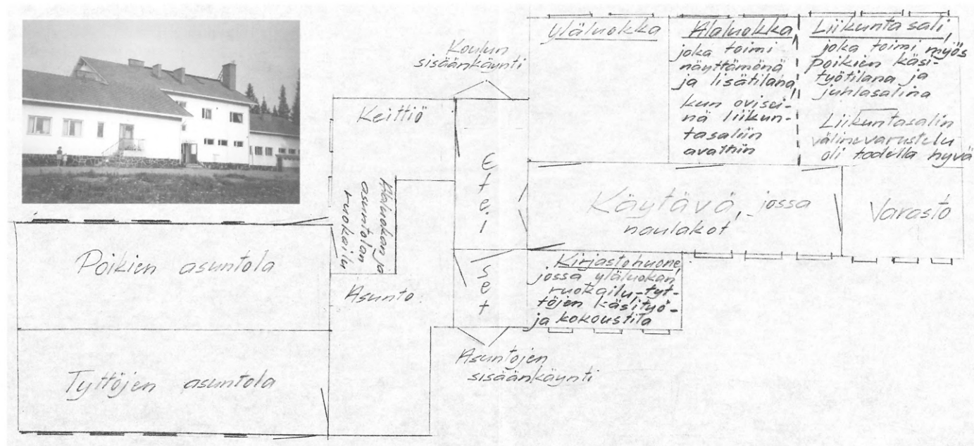
Uusi koulu ja sen pohjapiirros
