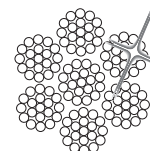
6x19+IWS
