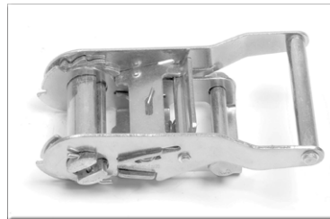
Tuotekoodi: SVKI1500 LC 1250 daN, 35 mm nauhalle
