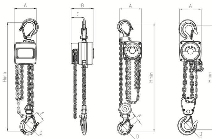
250 kg talja on erittäin pienikokoinen ja kevyt käyttää
