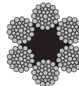
6x36+FC
