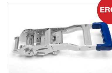
Tuotekoodi: SVKI2035ERGO LC 2500 daN, 50 mm nauhalle Ergo, alaspäin kiristävä
