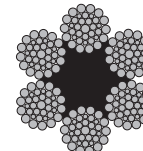
6x36+FC
