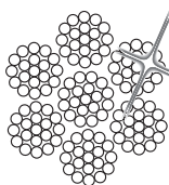
6x19+IWS
