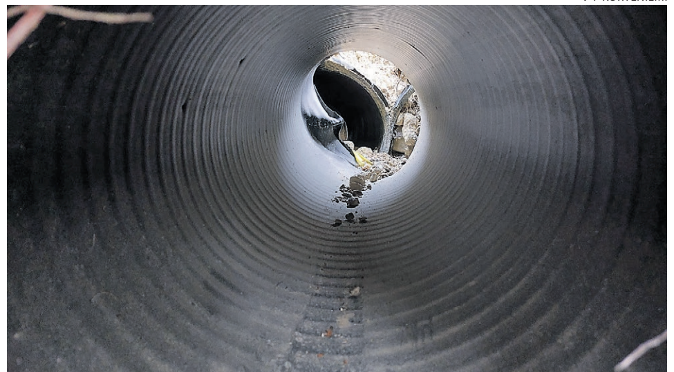
Kuva katkaistun rummun päästä: sovittu asennuksesta sisäluiskaan, mutta aura-asennus on tehty keskelle tietä.
